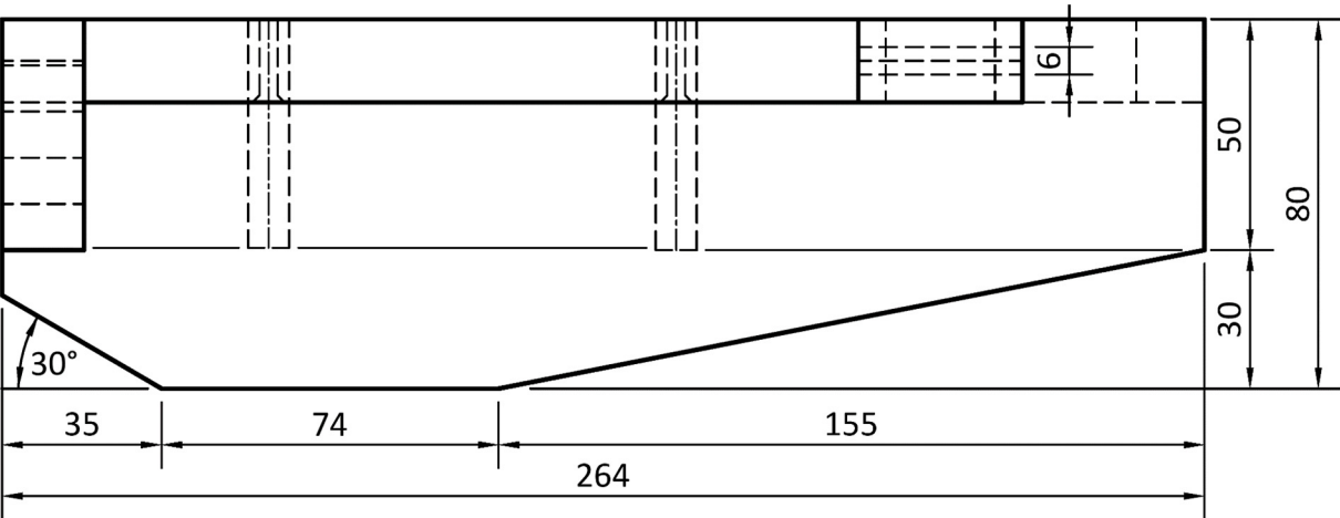
Plan/Bonnchló
